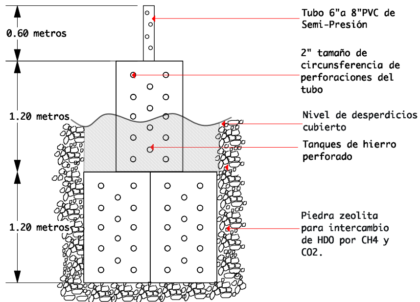
Vista en elevación de estructura para desfogue
