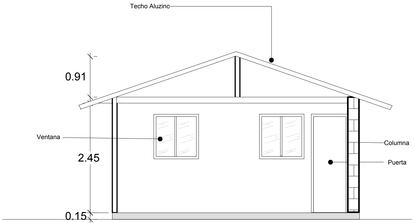
Elevación Frontal Esc: 1:50
