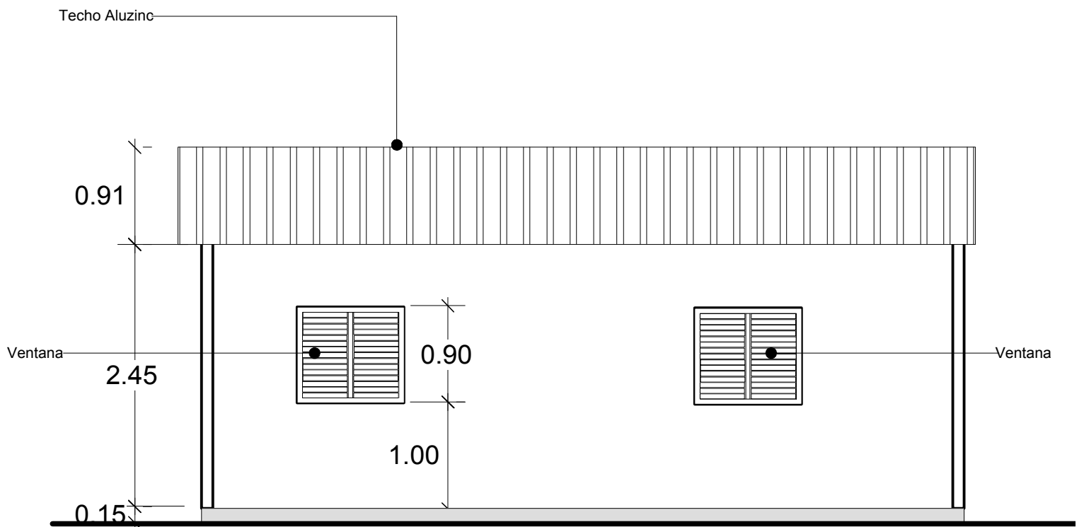
Elevación Lat. Izquierdo Esc: 1:50
