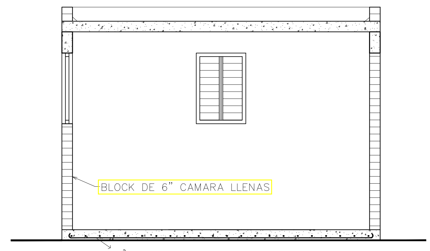
SECCIÓN A-A' CUARTO DE MÁQUINA
