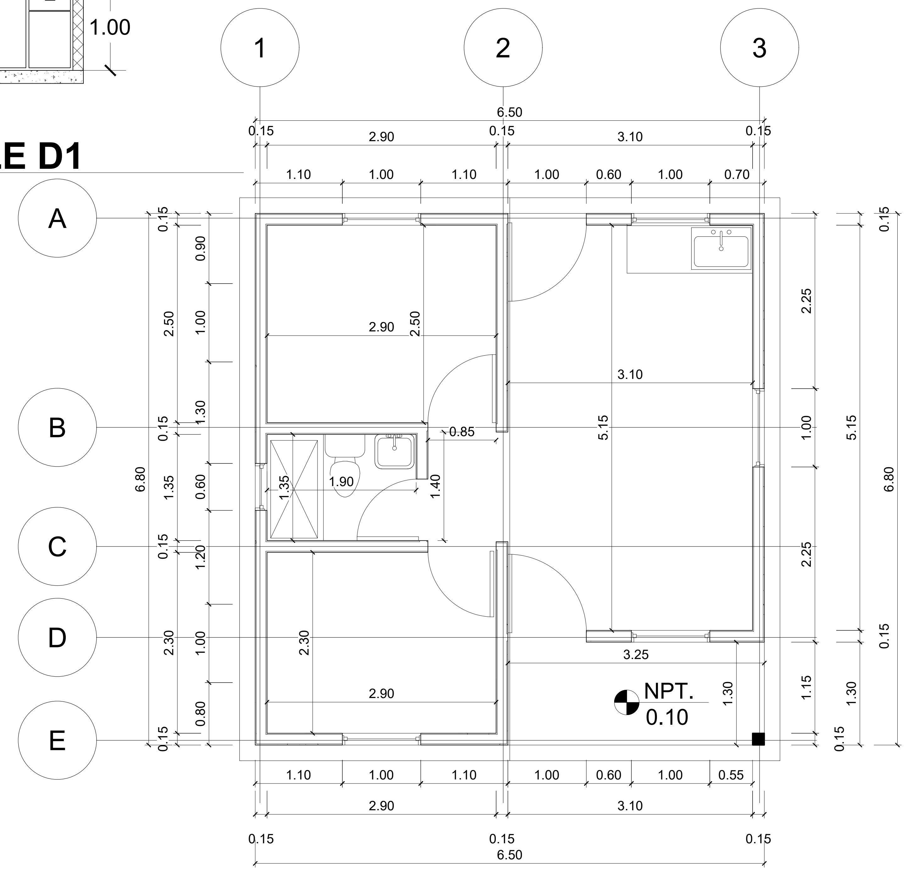
2 Planta Arq. Dimensionada 1 : 50
