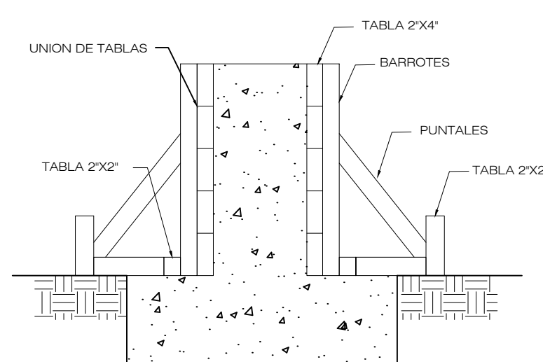
3 DETALLES TÍPICO DE ENCOFRADO DE MURO E-5 NO ESC.
