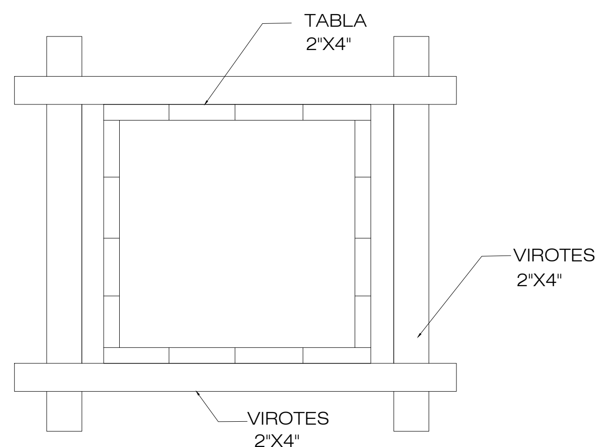
5 DETALLES TÍPICO DE ENCOFRADO DE COLUMNA E-5 NO ESC.
