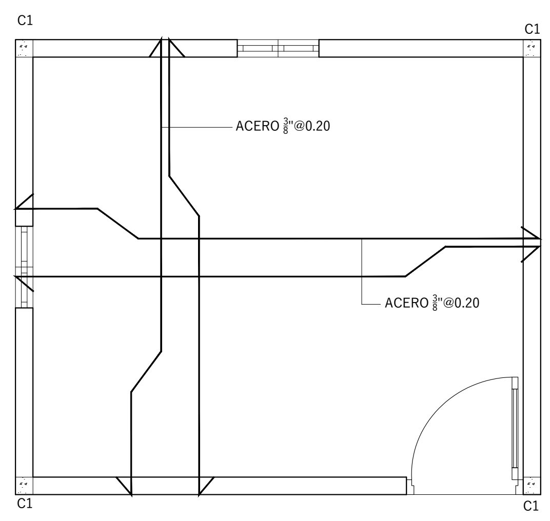
PLANTA CUARTO DE MÁQUINA
