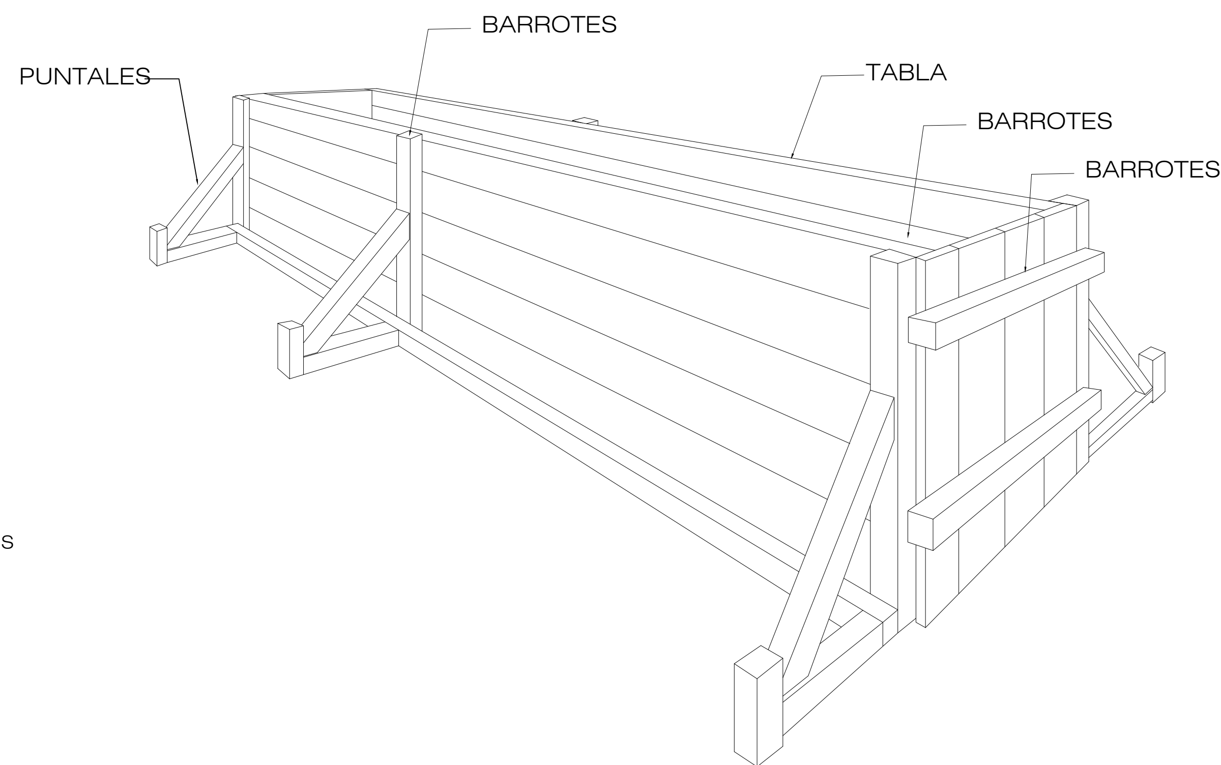
8 PERSPECTIVA ENCOFRADO DE MURO E-5 NO ESC.
