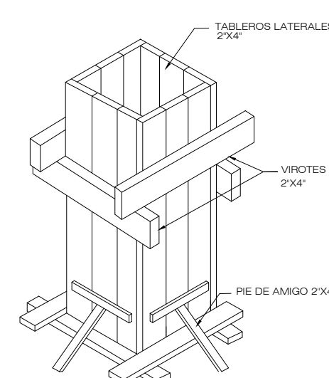
2 PERSPECTIVA ENCOFRADO DE COLUMNA E-5 NO ESC.
