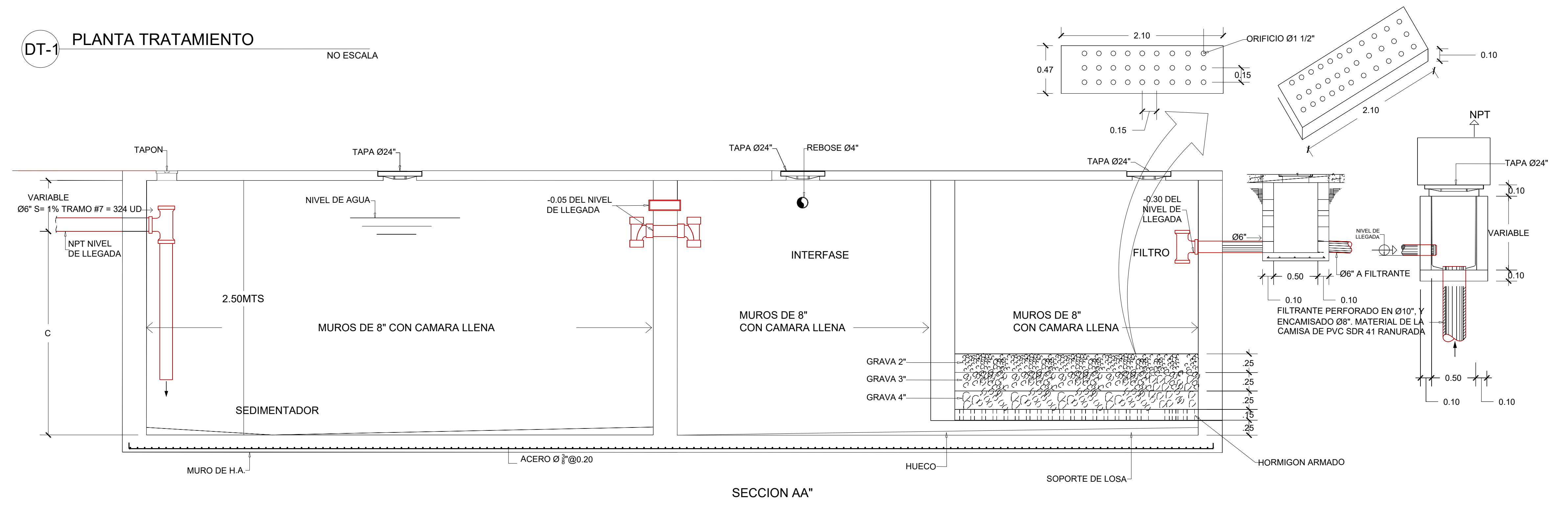
DT-1 SECCIÓN DE PLANTA TRATAMIENTO NO ESCALA
