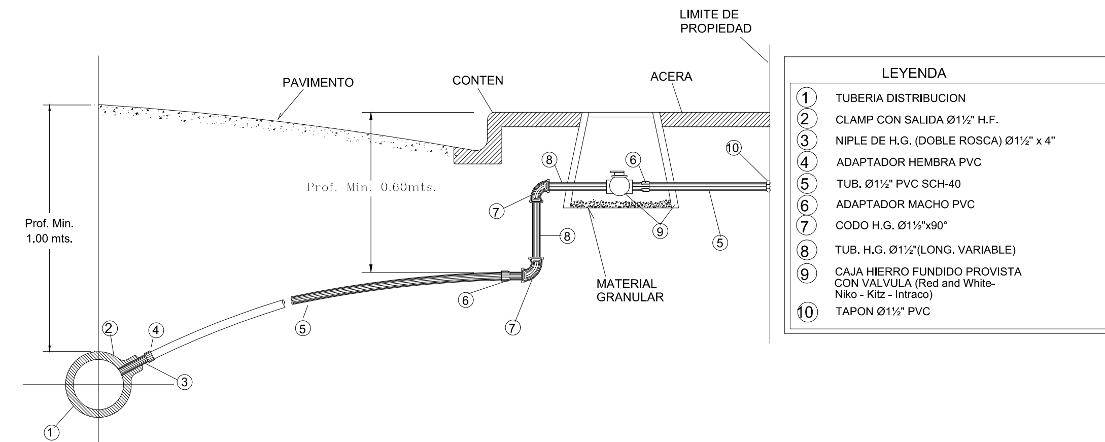
DT-3 DETALLE #3 CONEXION A ACOMETIDA TIIPICA NO ESCALA
