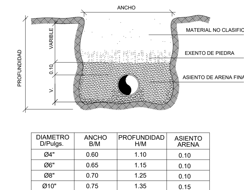
DT-6 DETALLE #6 EXCAVACION TIIPICA NO ESCALA
