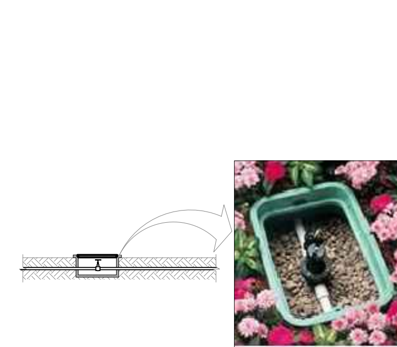
DT-4 DETALLE #4 CAJA DE VALVULAS NO ESCALA
