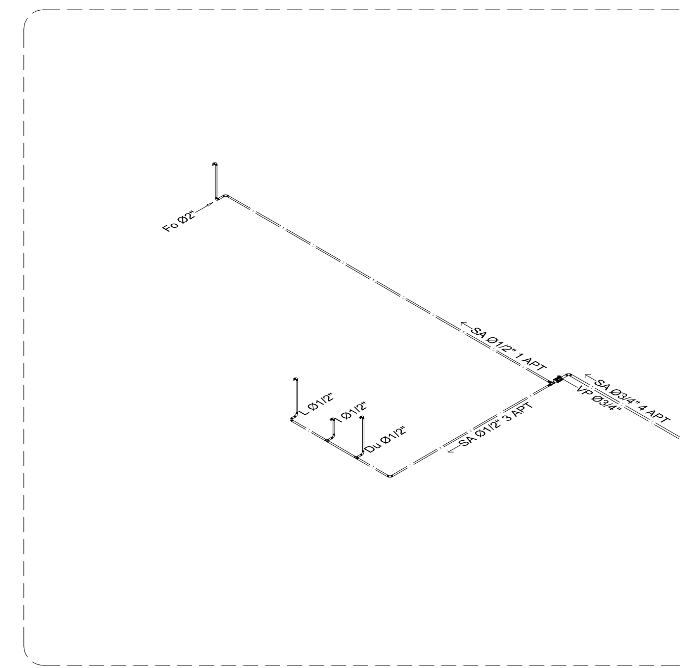
DT-2 ISOMETRICA SUMINISTRO DE AGUA VIVIENDAS EL SEIBO ESCALA 1:50
