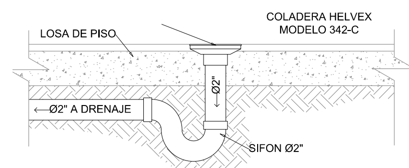
DT-7 DETALLE #7 DESAGUE DE PISO NO ESCALA
