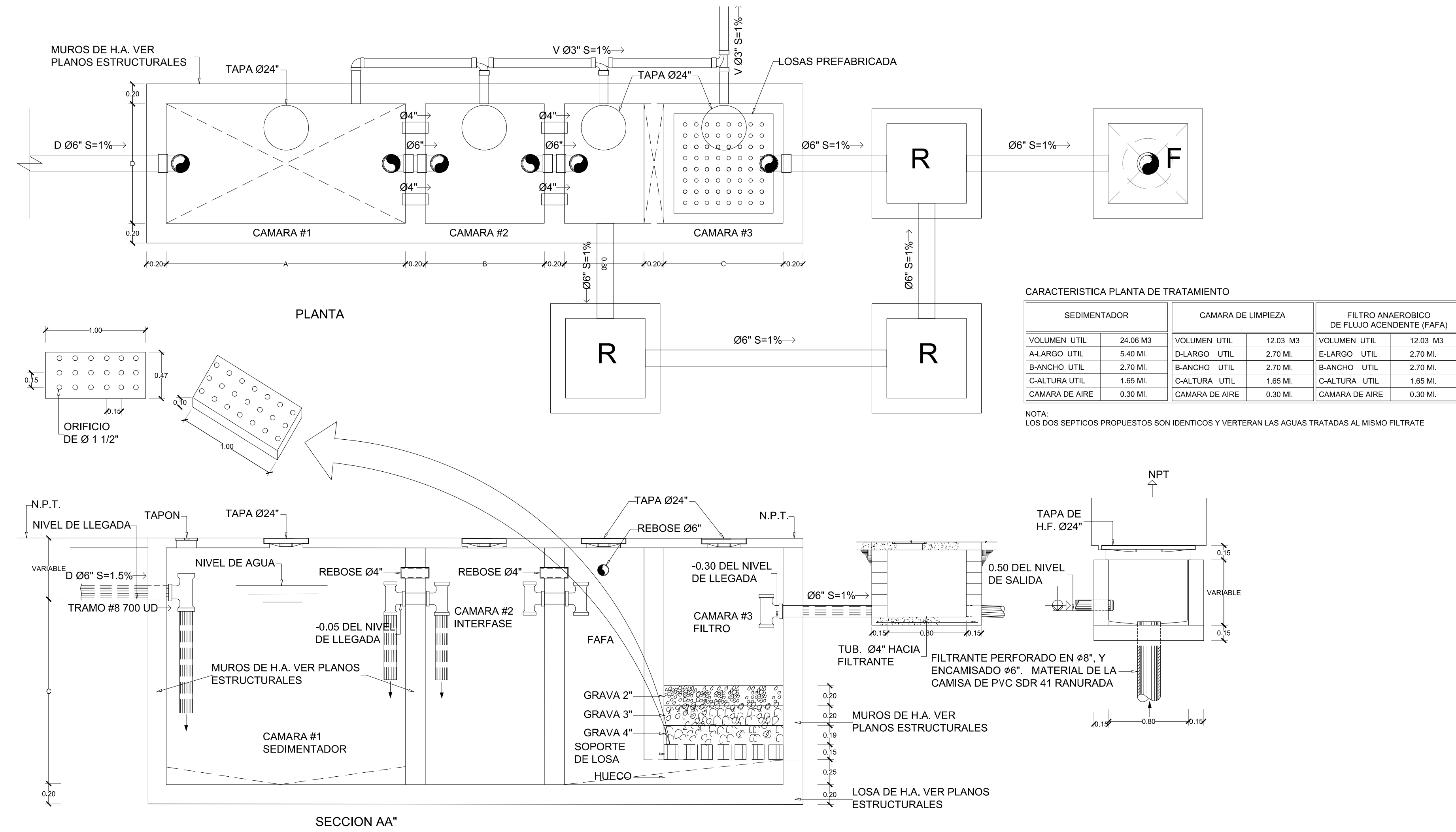
DT-1 DETALLE #1 SEPTICO (PLANTA DE TRATAMIENTO) ESCALA 1:30
