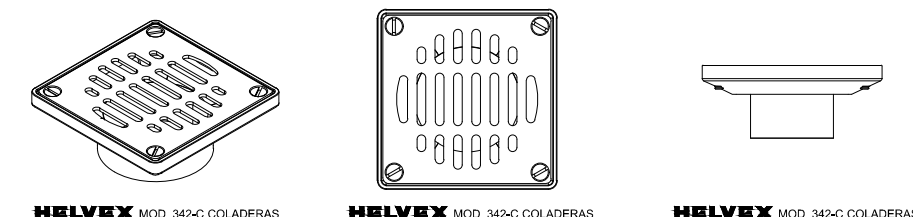
DT-8 DETALLE #8 REJILLA DE PISO HELVEX 342-C NO ESCALA
