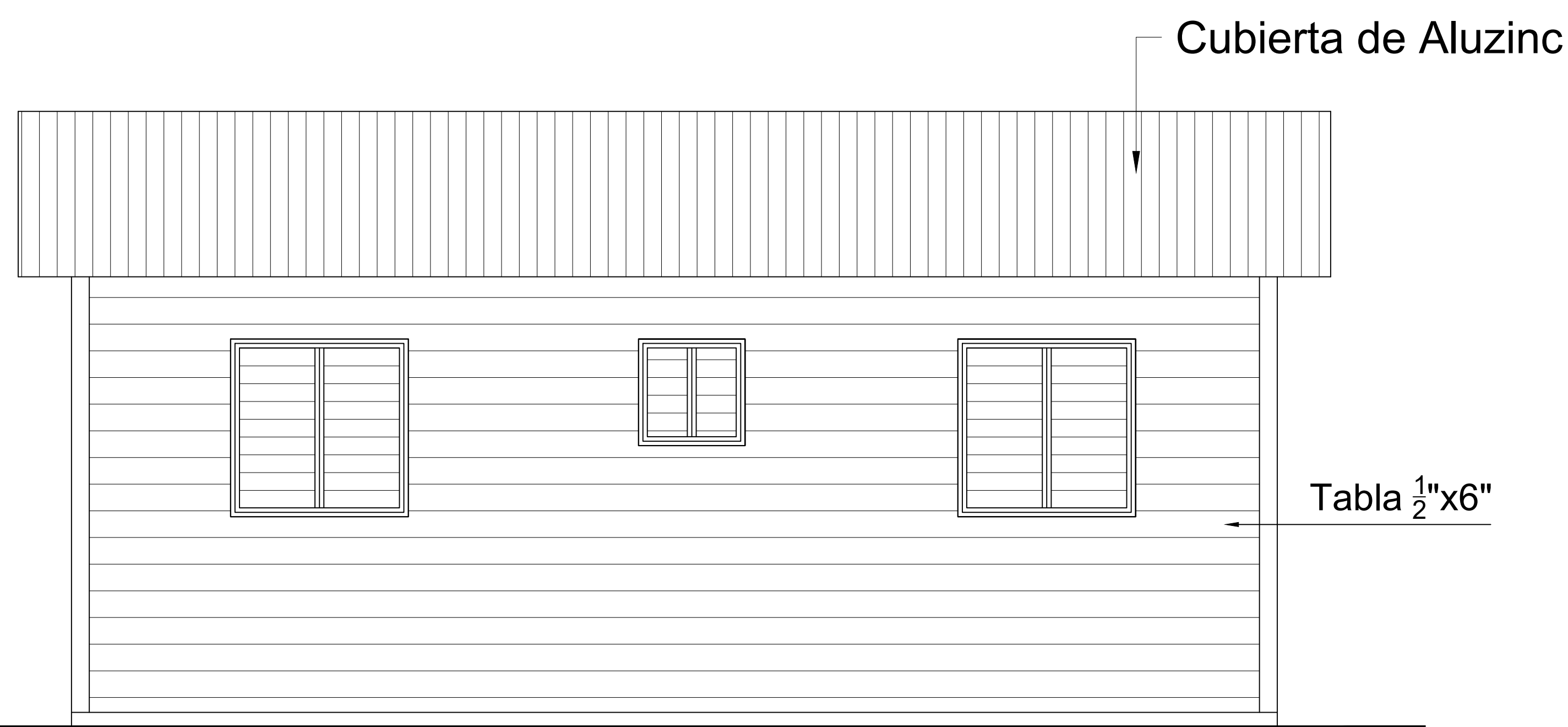
1 ELEVACIÓN POSTERIOR
