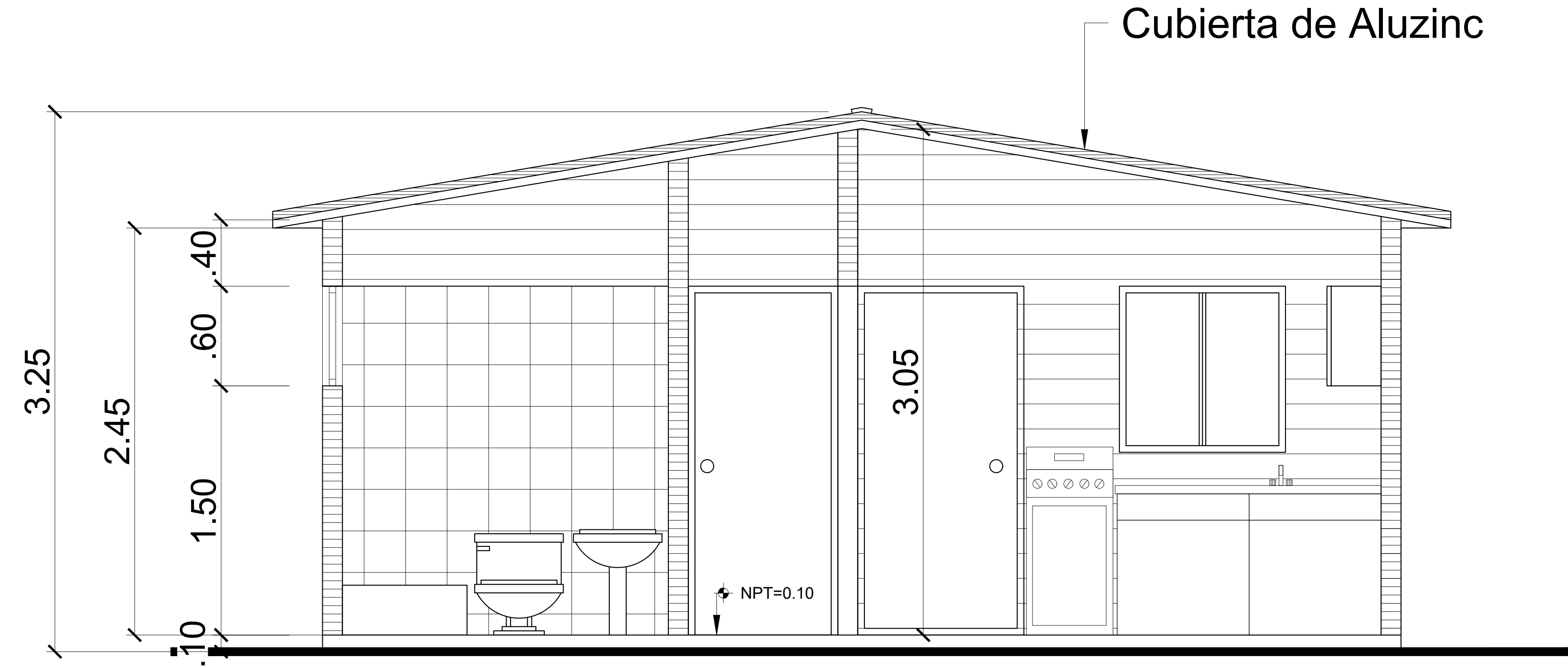
1 SECCIÓN A-A
