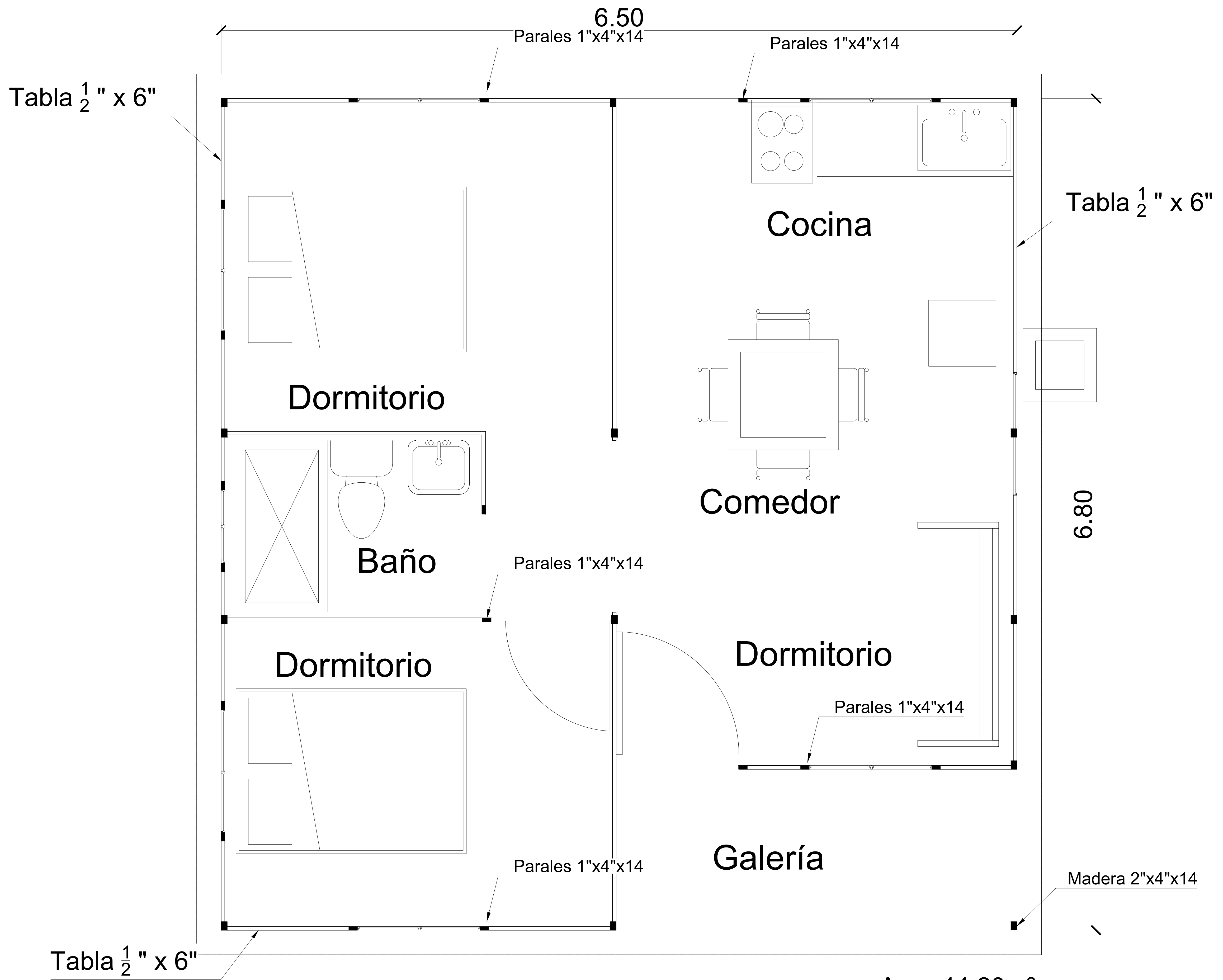
1 Planta Arquitectónica
