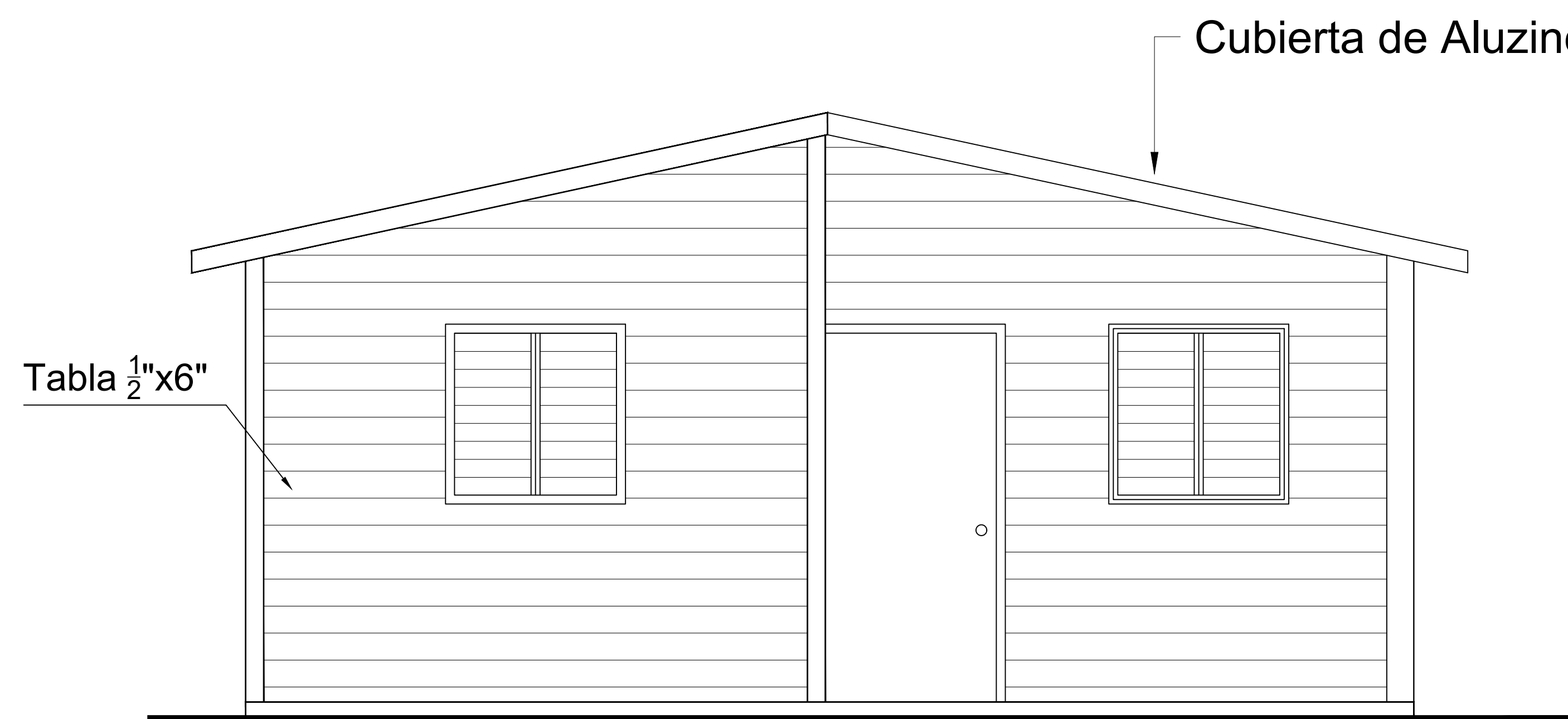
1 ELEVACIÓN FRONTAL
