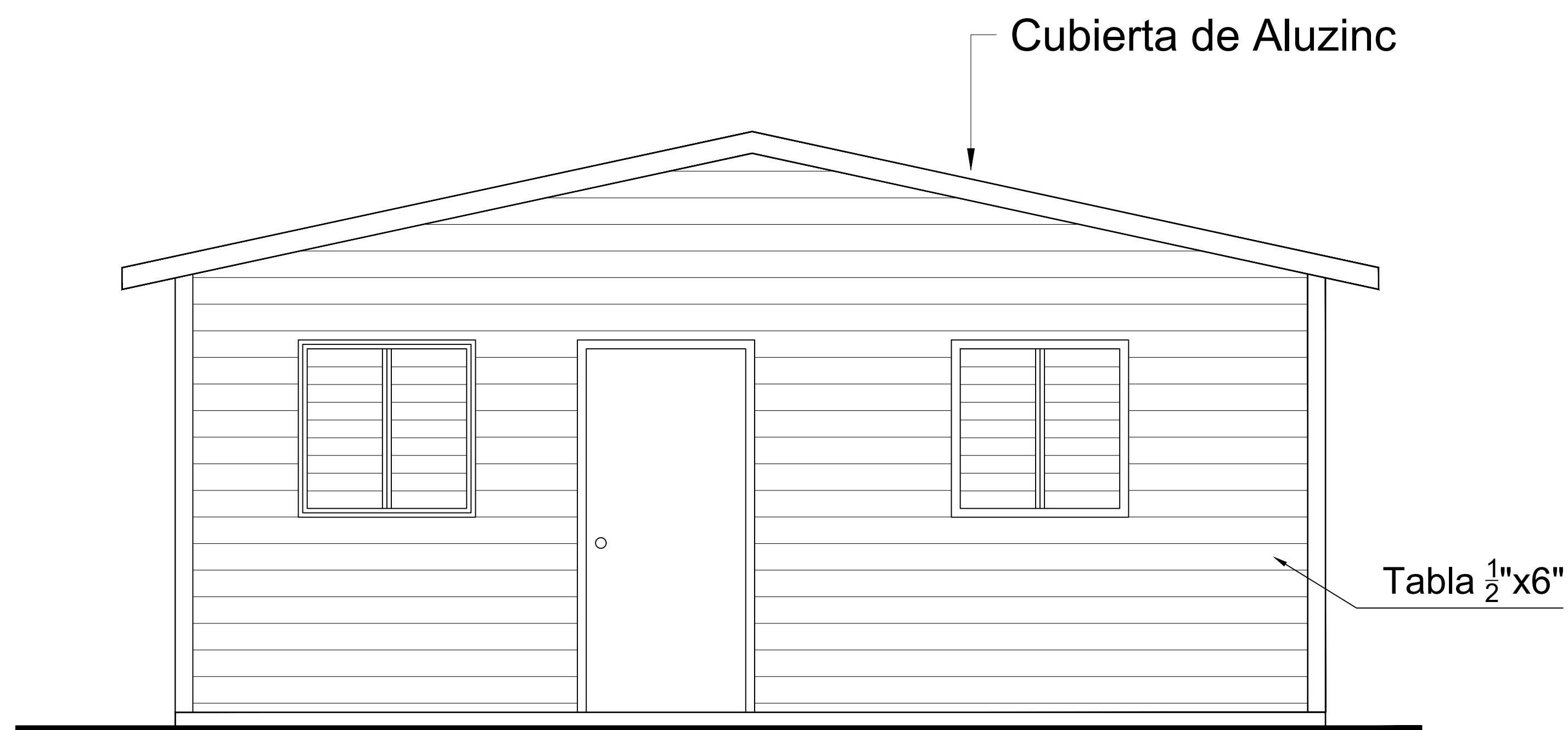
1 ELEVACIÓN POSTERIOR
