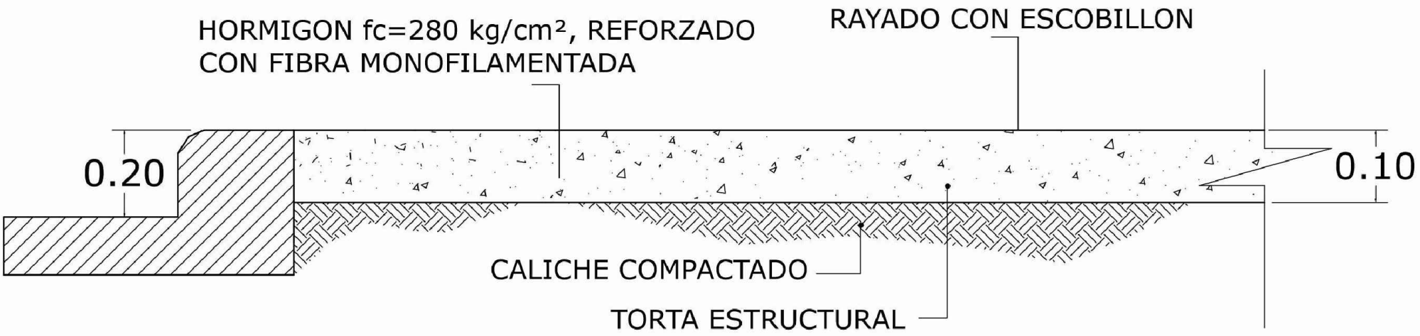
SECCION TRANSVERSAL
