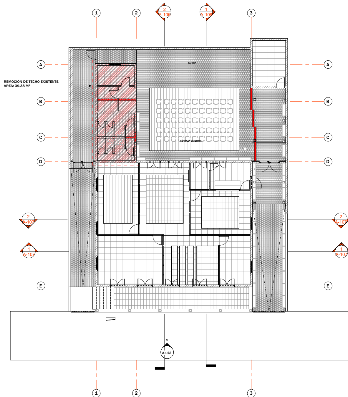
1 PLANTA DE DEMOLICION SCALE: 1:100
