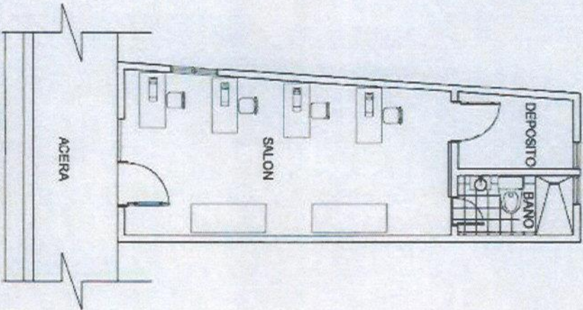
PLANTA ARQUITECTONICA AMUEBLADA
